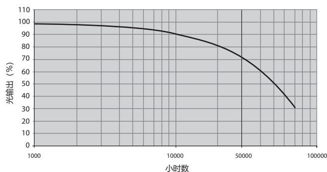
图1：光量与时间预计关系图
