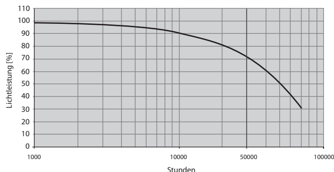
Kurve 1: Geschätzte Lichtleistung im Laufe der Zeit
